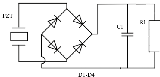
9 pav. Elektrinė kinetinės energijos surinkimo schema: PZT – pjezoelektrinis keitklis; D1-D4 – įtampos lyginimo diodai; C1 – kondensatorius; R1 – elektrinė apkrova
